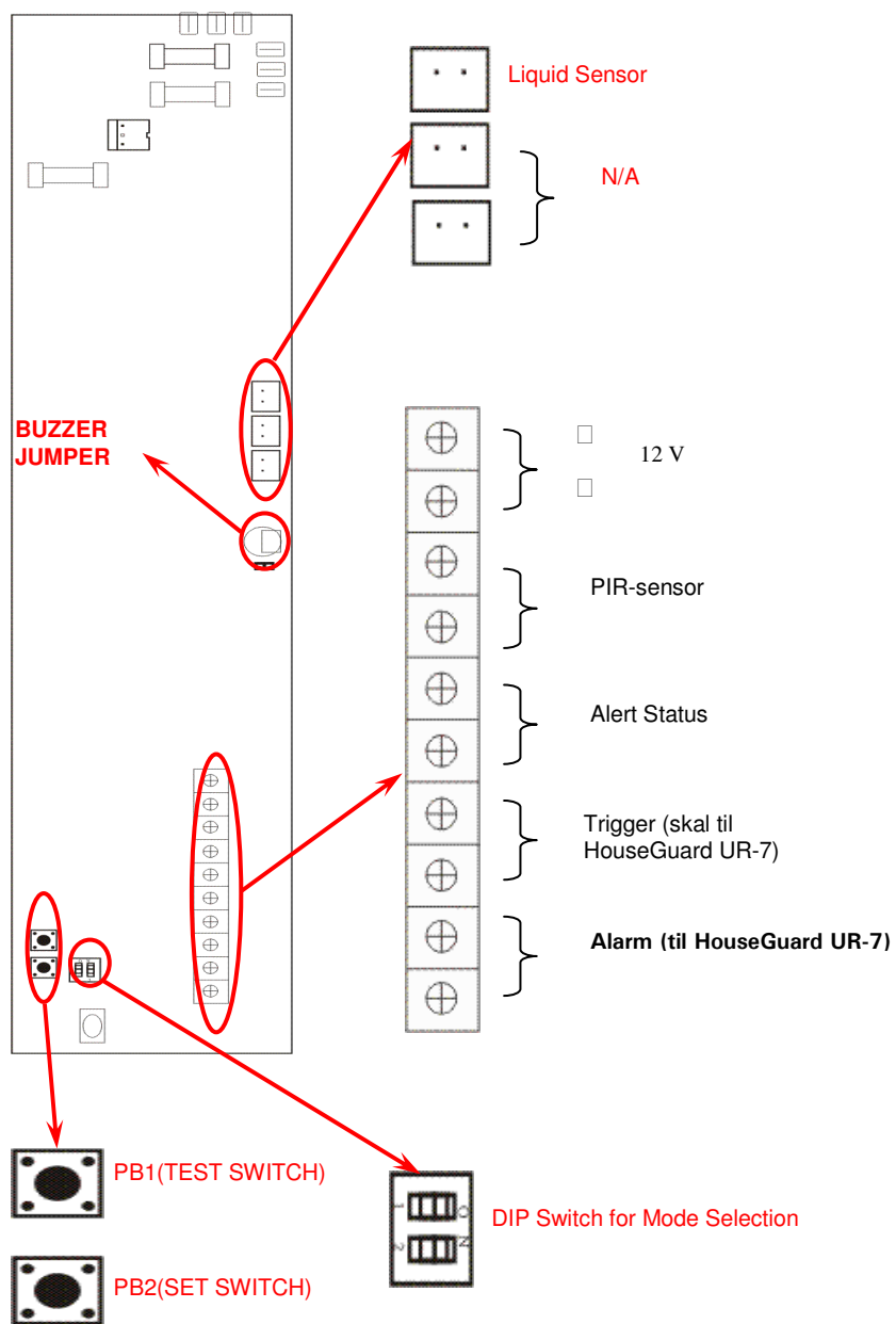
Oversigt over røgkanonens styringsprintplade. Kablet fra UR-7-relæet skal forbindes til både 'Trigger'- og 'Alarm'-terminalerne.
