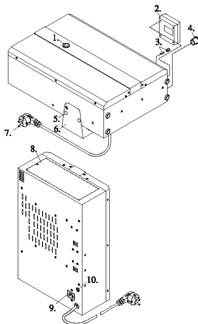
Oversigt over Røgkanon
